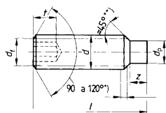
DIN 915 punta cilindrica with dog point
