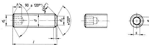
DIN 916 punta coppa with cup point
